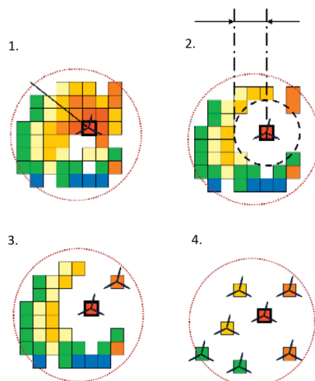
Abbildung 1-2: Methodik zur Standortwahl für WEA in Anlehnung an /IWES-02 11/
