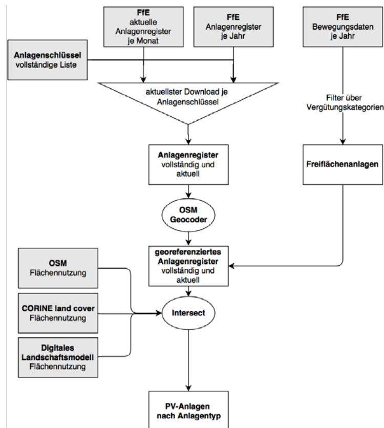
Abbildung 2-2: Aufbereitung der Anlagenregister in der EEGDB
