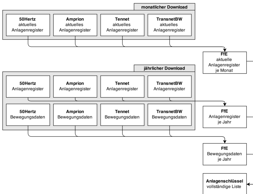
Abbildung 2-1: Zusammenführung der Quellen in der EEGDB bis Juli 2014.
