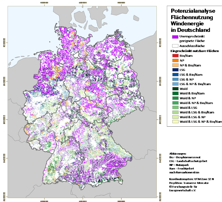
Abbildung 1-6: Uneingeschränkt und eingeschränkt nutzbare Flächen für Windenergie in Deutschland /KLI-01 14/
