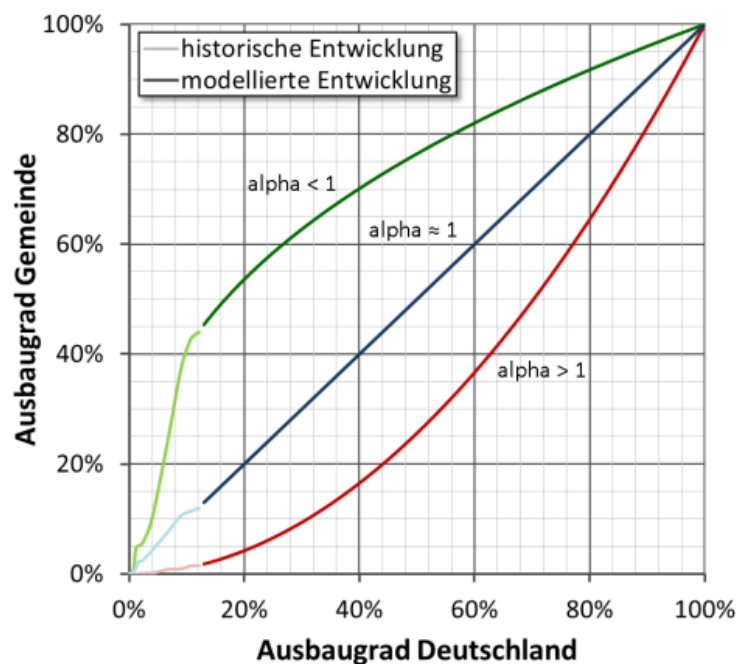
Abbildung 2-5: Bestimmung des Parameters Alpha für drei ausgewählte Gemeinden
