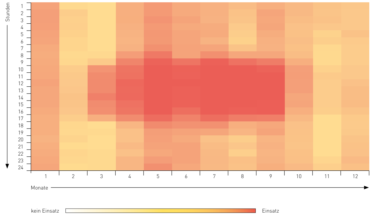
Abbildung 29: Einsatz last- und erzeugungsseitiger Flexibilität – Elektrolyse
