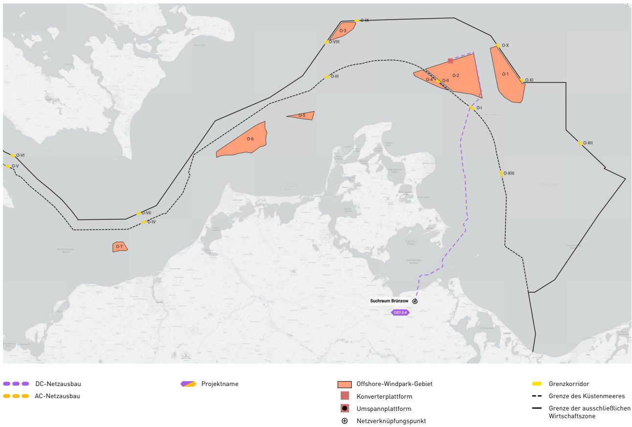
Abbildung 54: Maßnahmen des Offshore-Zubaunetzes der Ostsee in den Szenarien A / B / C 2037
