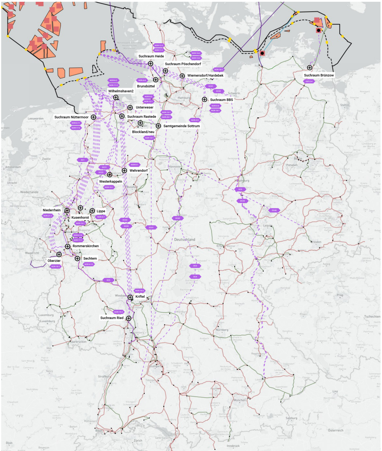
Abbildung 65: Mögliche Bündelung der neuen DC-Projekte und der Offshore-Anbindungssysteme in A/B/C 2045
