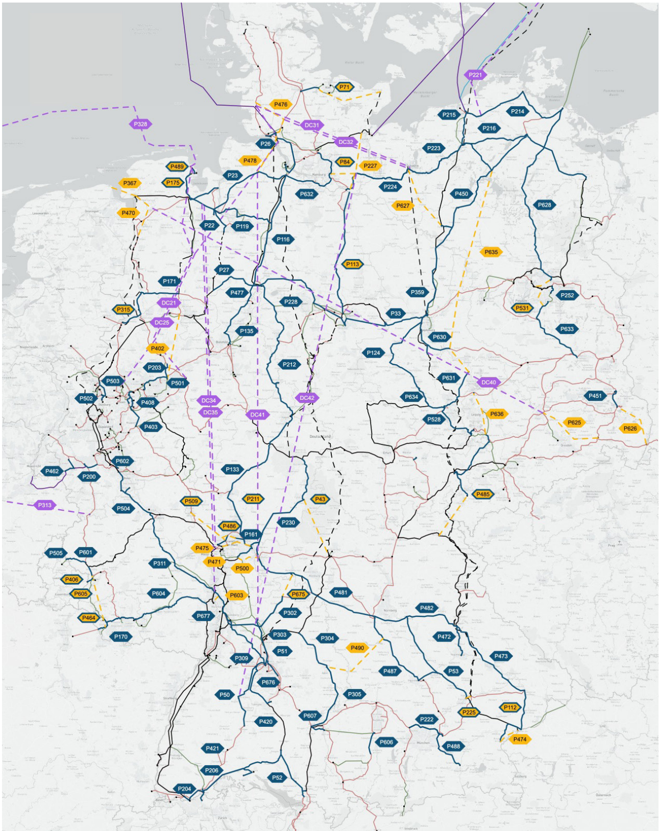
Abbildung 63: Szenario B 2037 / nur Leitungsprojekte*
