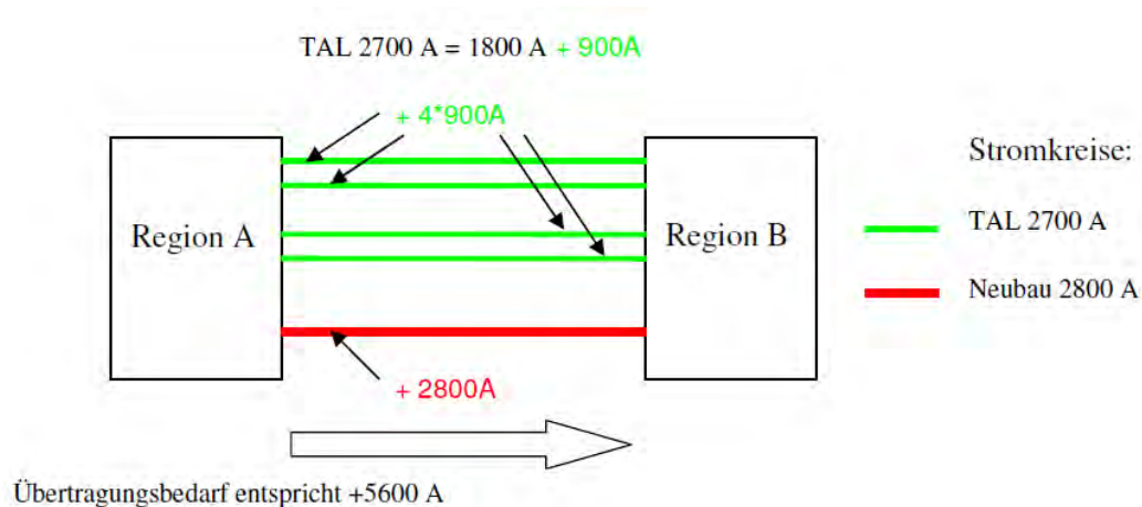
Abbildung 13-18: Modellnetz TAL1
