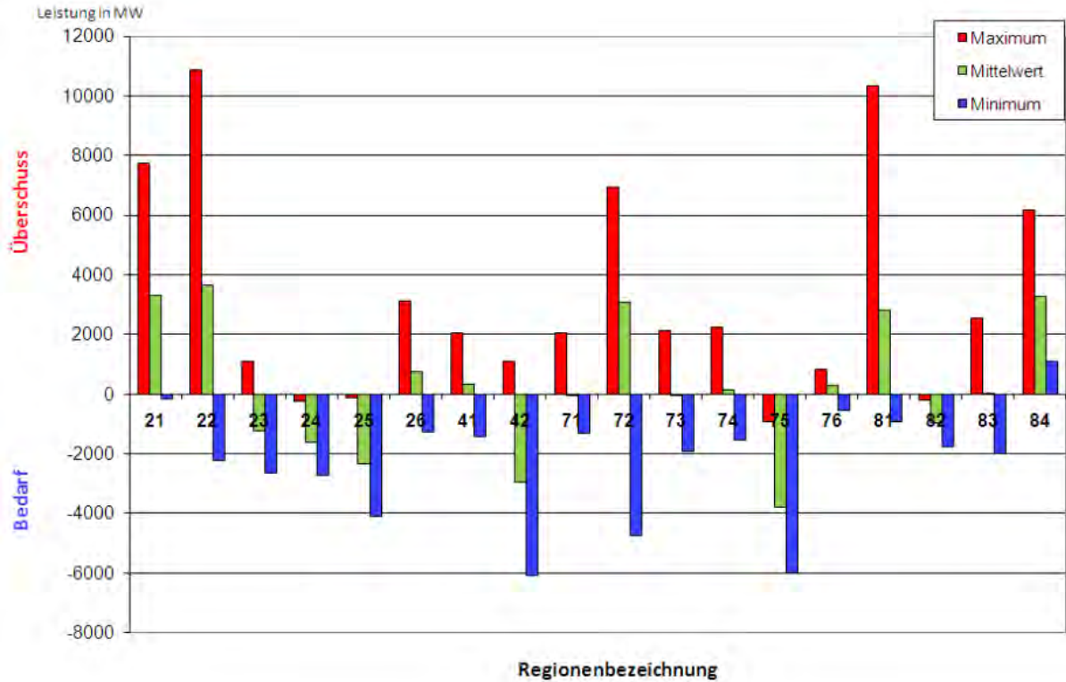
Abbildung 12-9: Regionenbilanz (Maximum, Minimum und Mittelwert je Region)
