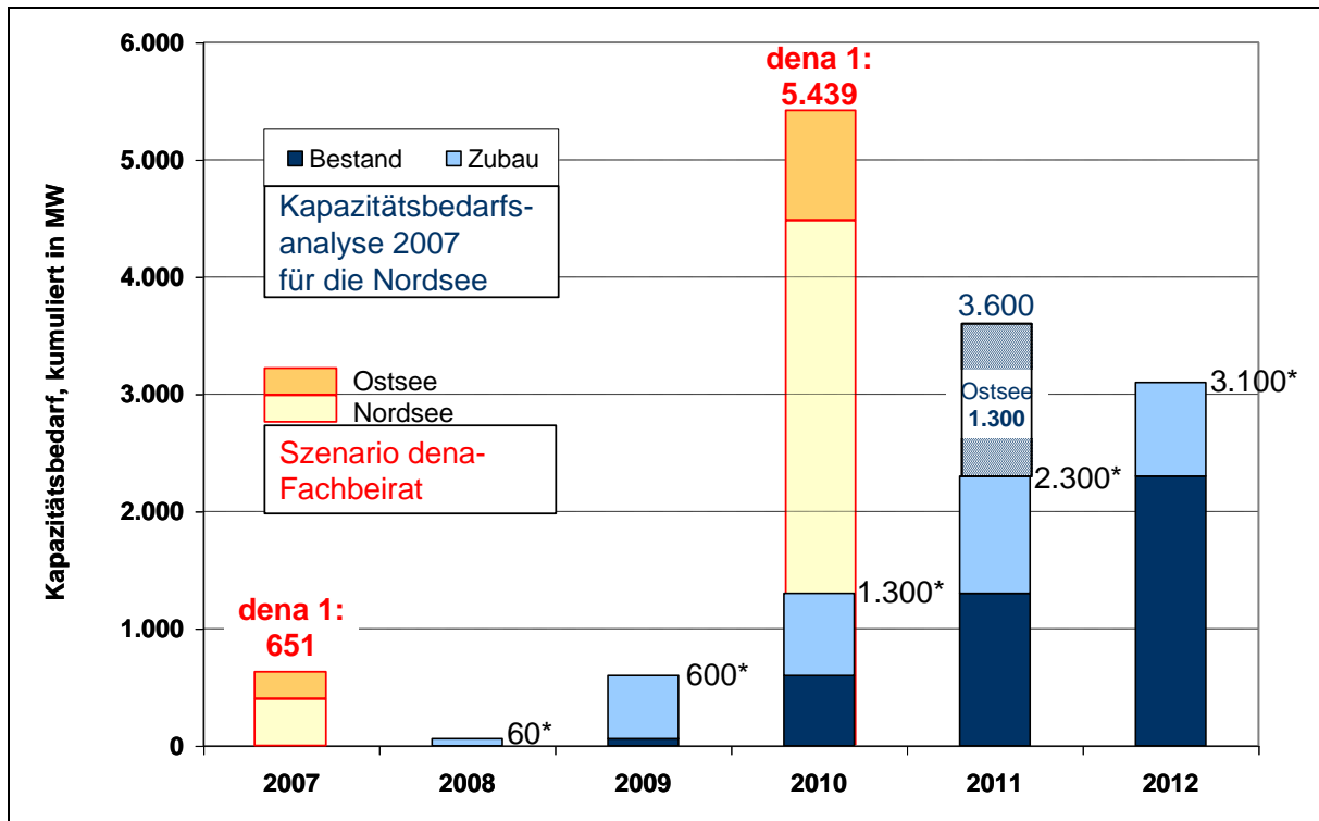
Abbildung 2-4: Offshore-Windenergieausbau gemäß „Szenario dena-Fachbeirat“ und gemäß Kapazitätsbedarfsabschätzung aus 2007
