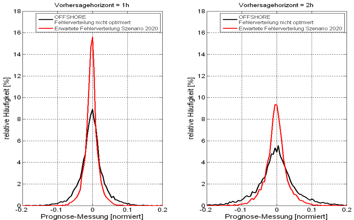
Abbildung 19-9: Fehlerverteilungen der nicht-optimierten und optimierten Windleistungsprognosen für Vorhersagehorizonte von ein (links) und zwei (rechts) Stunden für das gesamte Offshore Ausbauszenario 2020 normiert auf die Gesamtnennleistung von P_n=14070\text{MW}
