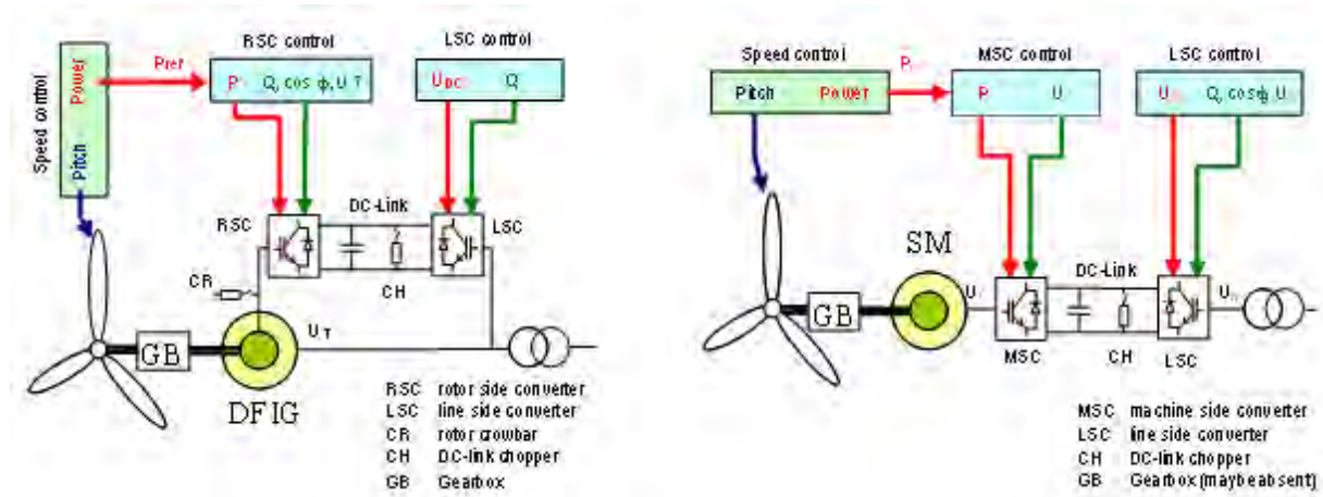
a) DFIG-Anlage
