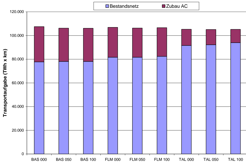
Abbildung 13-11: Überregionale Transportaufgabe des Übertragungsnetzes 2020
