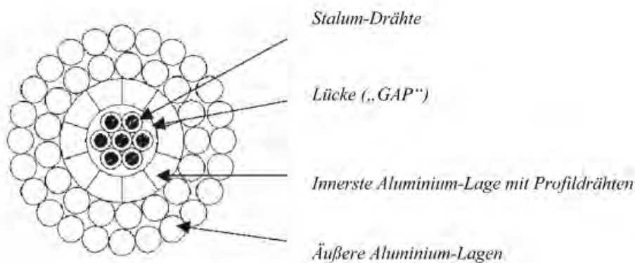
Abbildung 9-3: Aufbau eines GTACSR-Leiters
