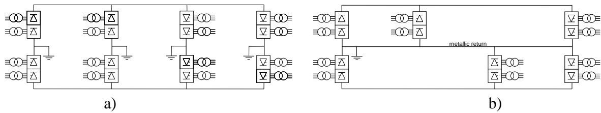
Abbildung 11-22: Klassische HGÜ als Multi-Terminal mit bipolarer (a) und hybrider (b) Ausführung
