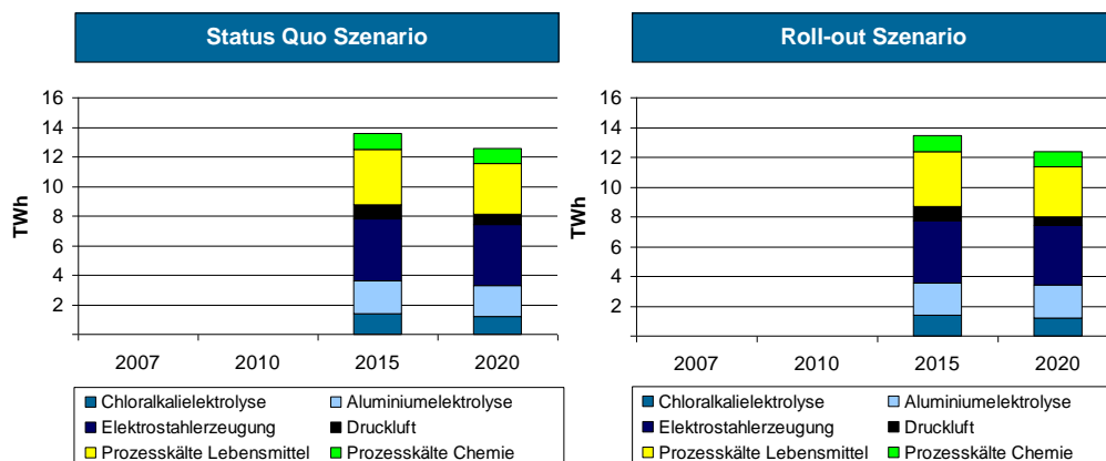
Abbildung B-0-14: Durch DSM verschobene Last im Industriesektor bis zum Jahr 2020
