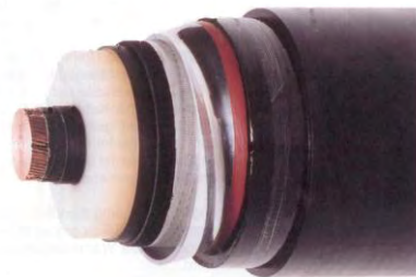
Abbildung 10-3: Querschnitt durch ein einadriges Höchstspannungsdrehstromkabel
