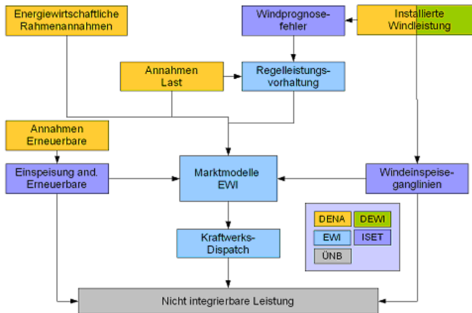
Abbildung 23-3: Arbeitsschritte zur Ermittlung der nicht integrierbaren Leistung
