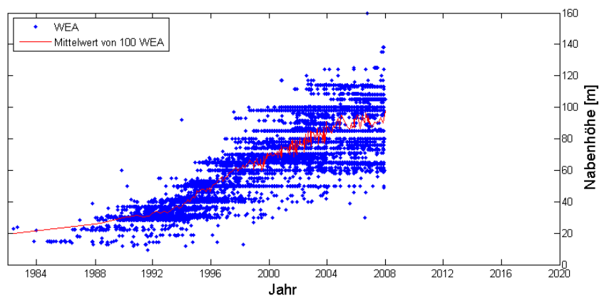
Abbildung 6-31: Nabhöhen aller bis 2008 errichteten WEA
