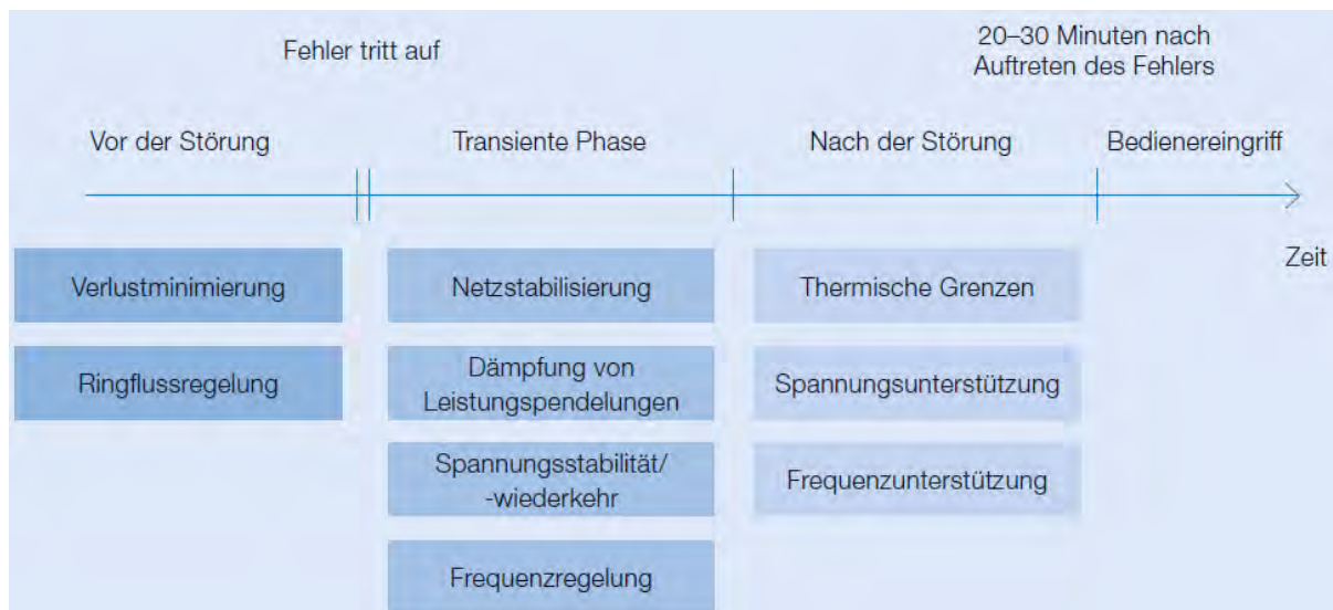
Abbildung 14-12: Erweiterte Regelungsstrategien der VSC-HGÜ
