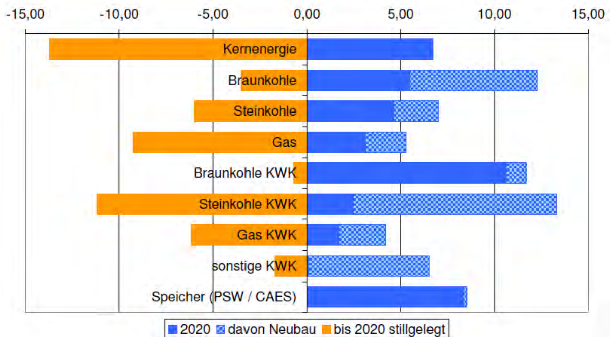
Abbildung E- 1: Kraftwerksentwicklung (in GW) bis zum Jahr 2020 im Basisszenario ohne Laufzeitverlängerung
