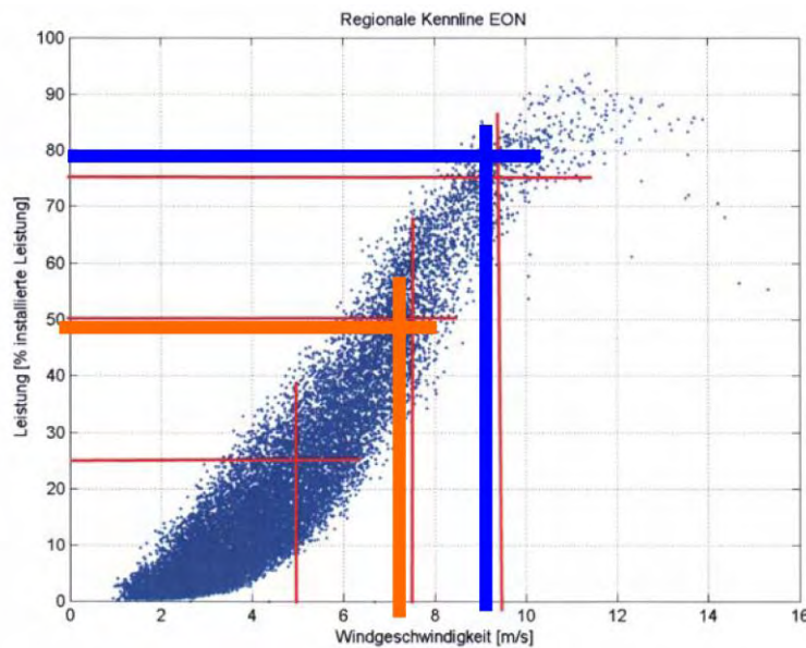
Abbildung 9-13: Windeinspeisekennlinie in der E.ON-Netz-Regelzone 2006-2007
