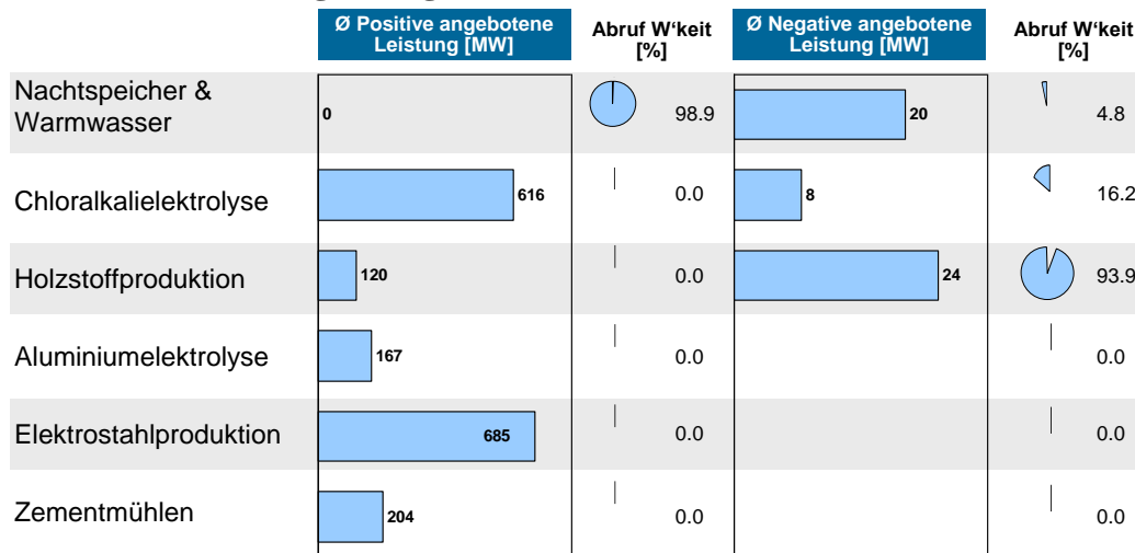
Abbildung 23-7: Dargebotene durchschnittliche Reserveleistung durch DSM Prozesse im Jahr 2020 sowie Wahrscheinlichkeiten für den Abruf von Regellenergie
