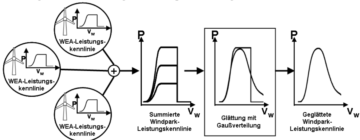
Abbildung 6-13: Erstellung einer Windpark-Leistungskennlinie
