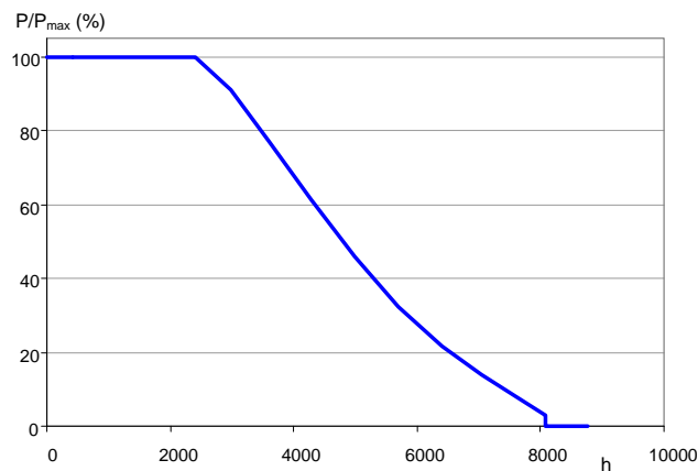
Abbildung 10-18: Typische Jahrgangskennlinie für Offshore-Windparks
