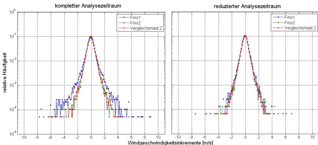
Abbildung 6-5: Häufigkeitsverteilung der Offshore Windgeschwindigkeitsinkremente
