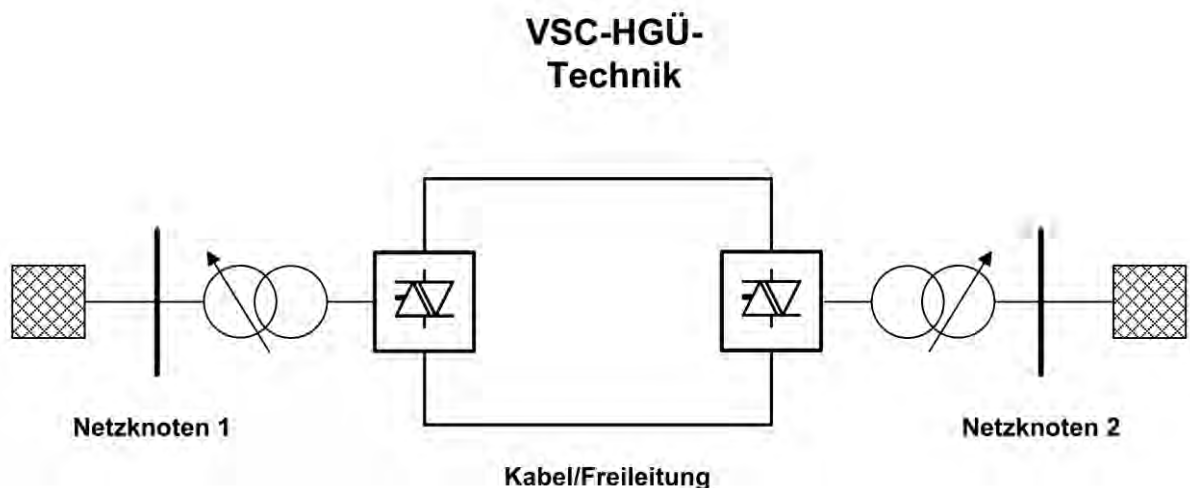
Abbildung 10-11: Schematische Darstellung einer Übertragung mit VSC-HGÜ-Technologie
